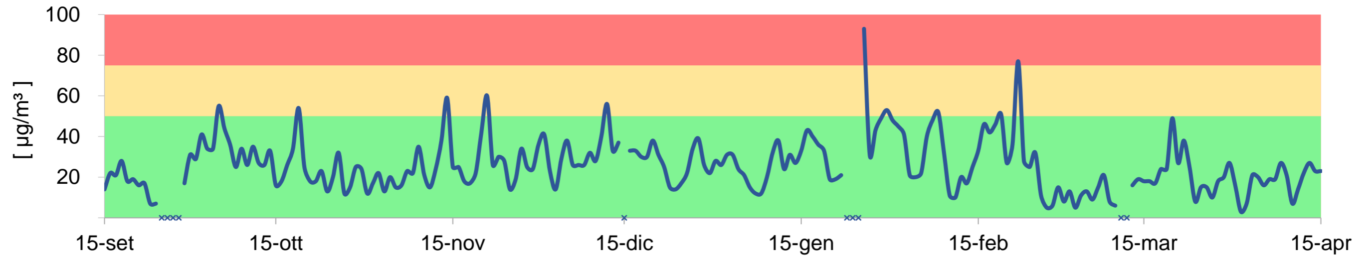
Figura 1: Valori di particolato PM 10 misurati dagli strumenti automatici del SRRQA
